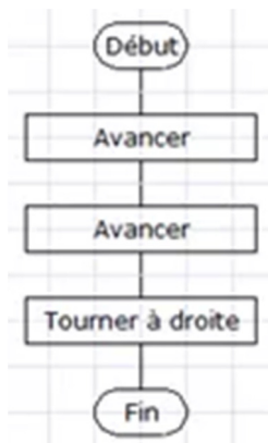
Sous-programme : AvancerDroite
