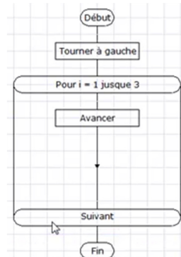
Sous-programme : AvancerGauche
