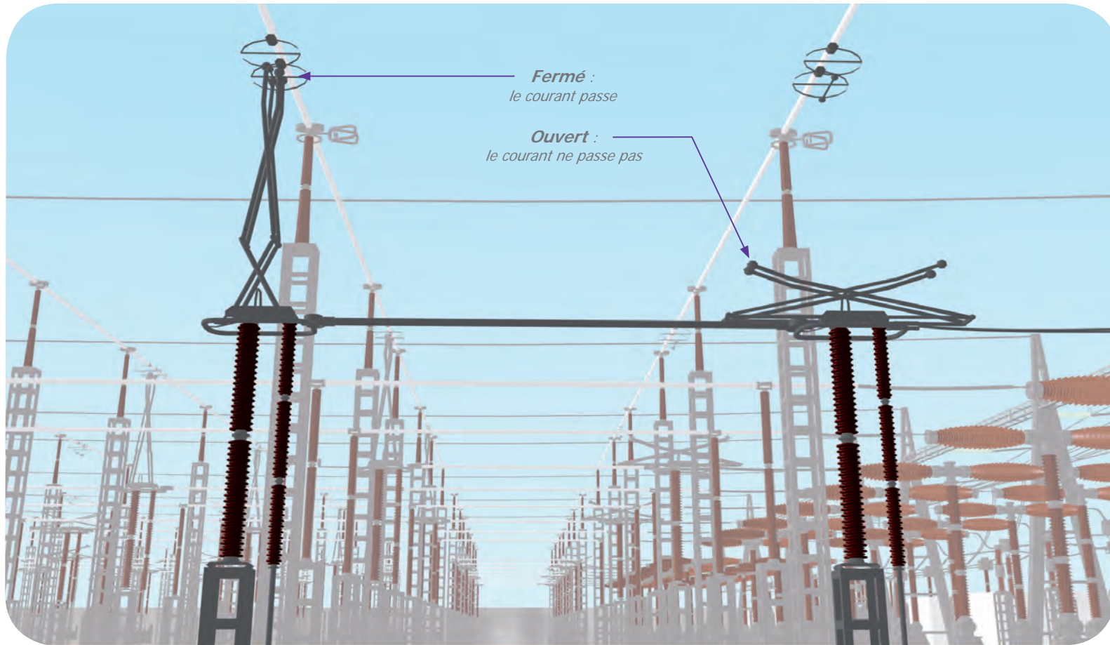
Sectionneur d'aiguillage
